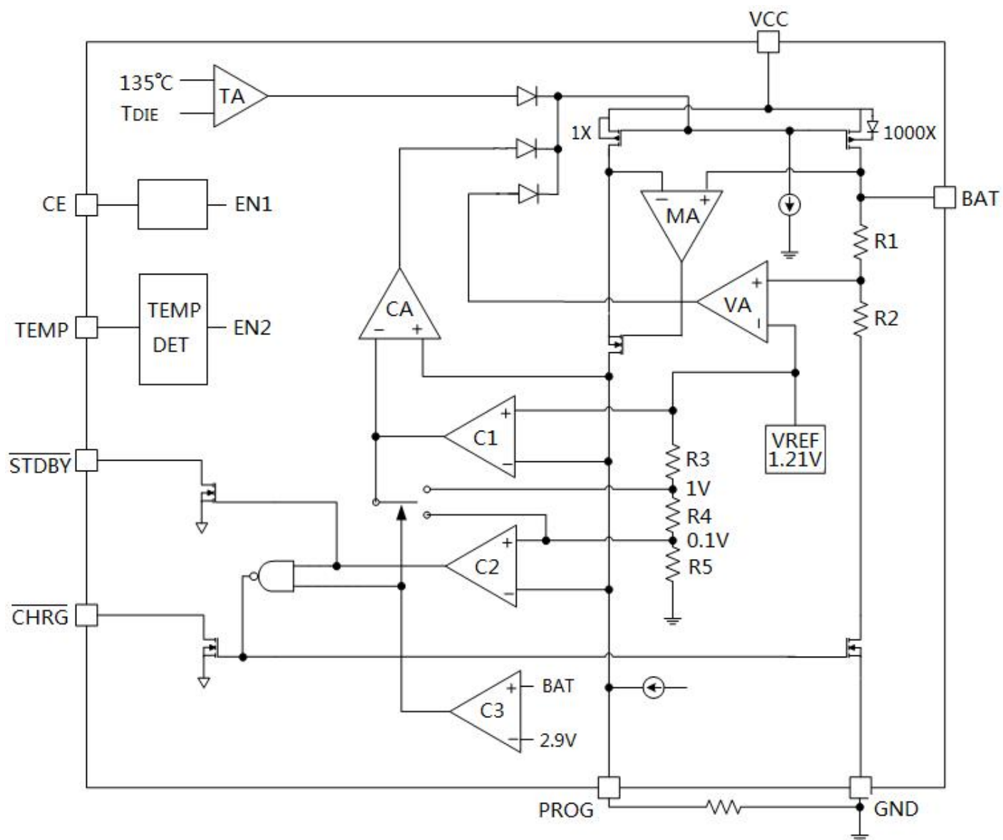
结构框图
