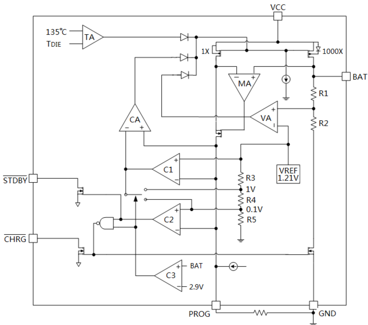
结构框图
