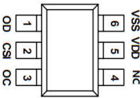
图 3 DW01AP 的 SOT23-6 封装及引脚排布
