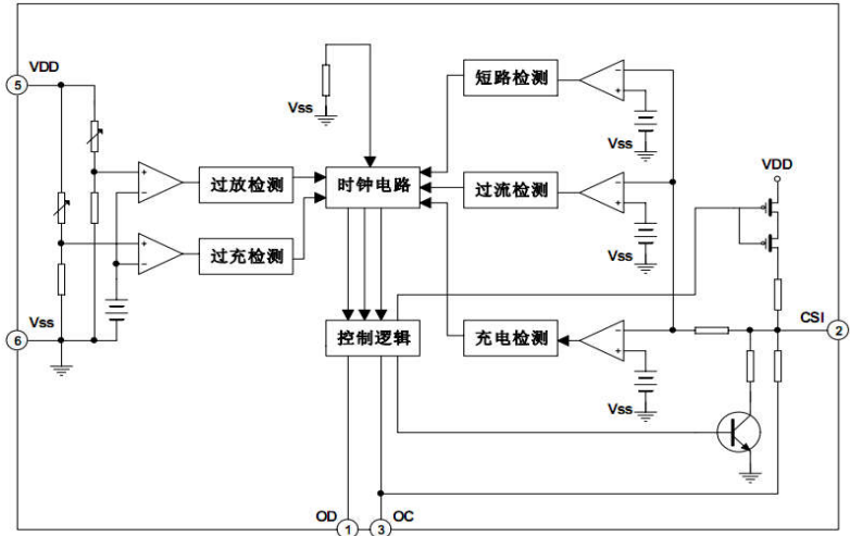
图2 功能框图
